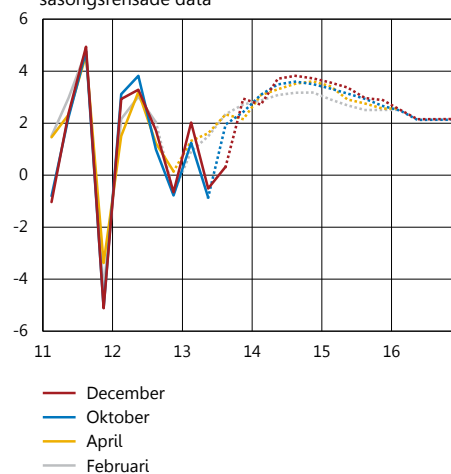
Diagram 3:1. BNP, prognoser 2013
