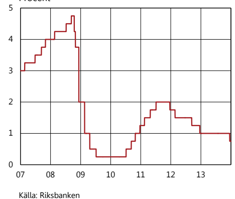
Diagram 1:8. Reporänta
