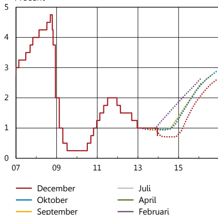
Diagram 3:3. Reporänta, prognoser 2013
