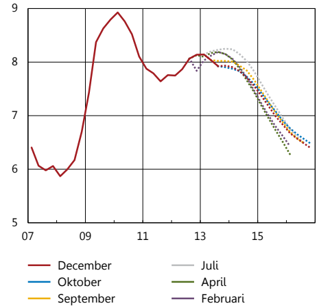
Diagram 3:12. Arbetslöshet, prognoser 2013
