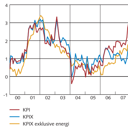
Diagram 9. KPI, KPIX och KPIX exklusive energi Årlig procentuell förändring
